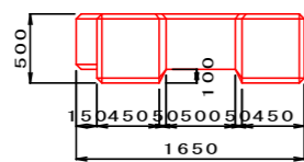
正面図
